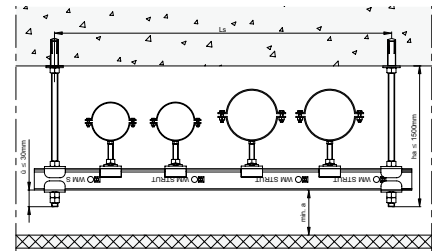
Konsolenkonstruktion
