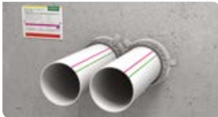
Nullabstand bei ungedämmten Rohren
