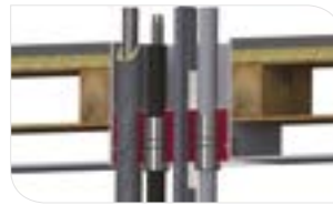
Holzbalkendecke (siehe S. 64)
